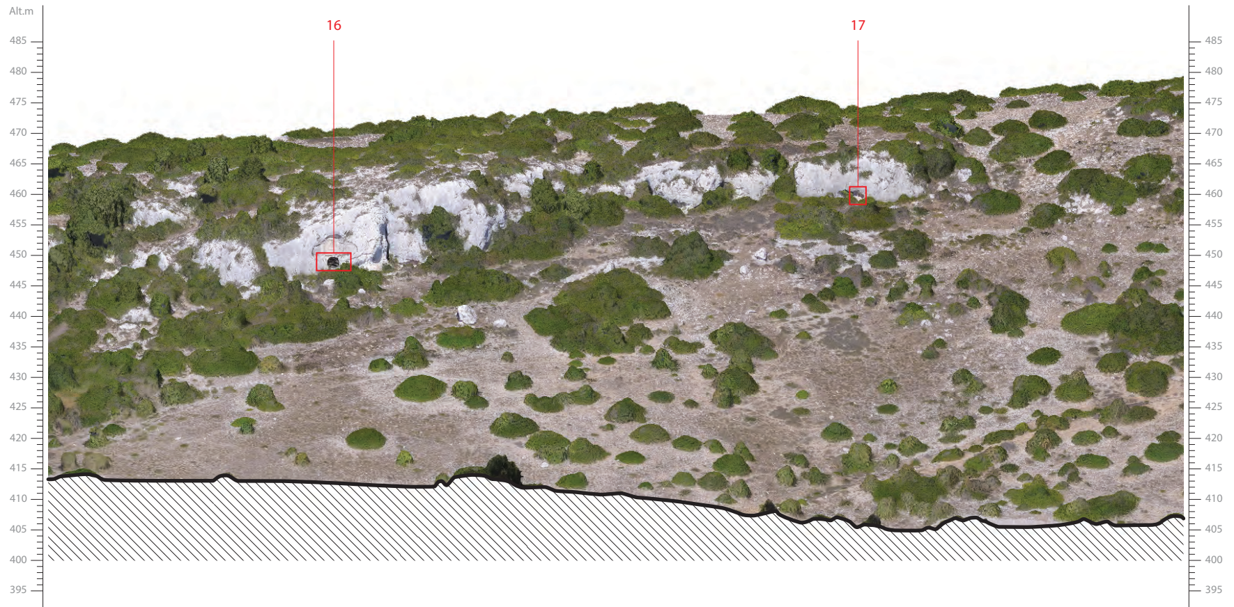
Ossi (SS) - Mesu 'e Montes Sector 2 (Domus 16-17) - ELEVATION
