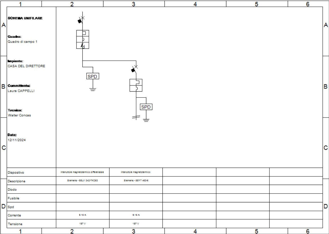
Fig. 8: Schema unifilare quadro "Quadro di campo 1"
