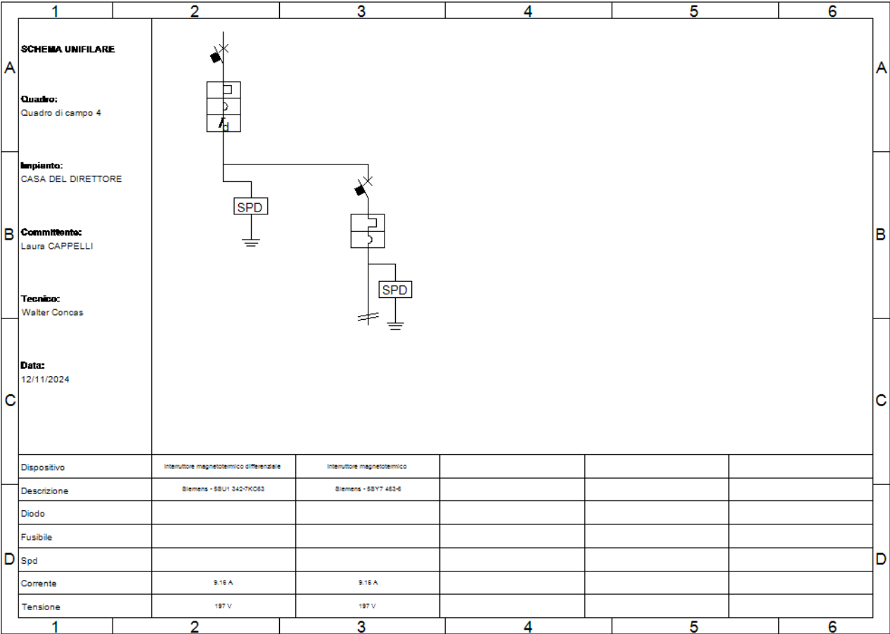
Fig. 12: Schema unifilare quadro "Quadro di campo 4"
