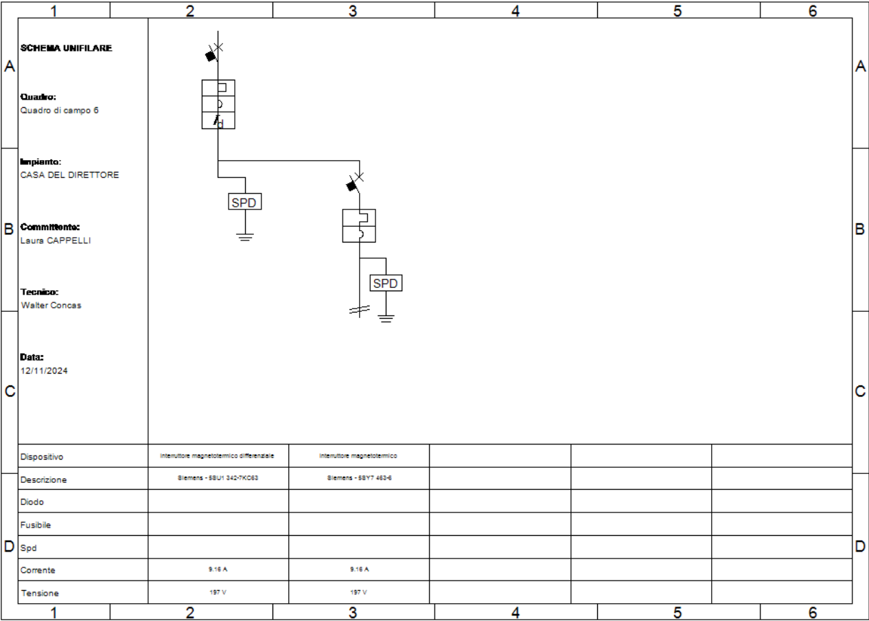
Fig. 15: Schema unifilare quadro "Quadro di campo 6"
