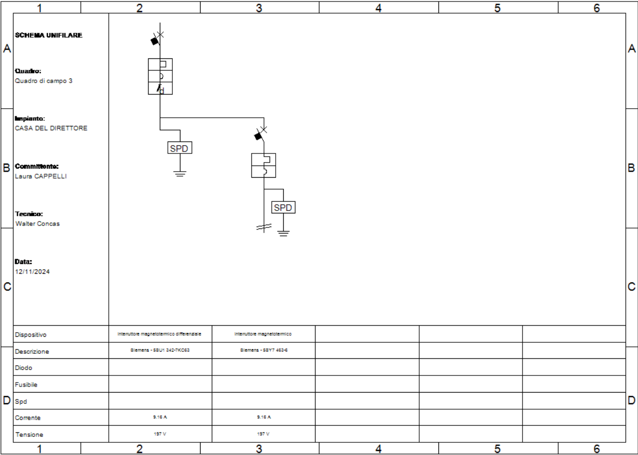
Fig. 11: Schema unifilare quadro "Quadro di campo 3"
